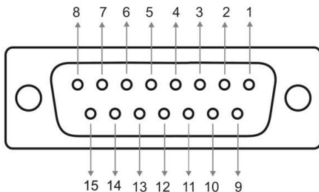
PC-Pro (DB15F)
