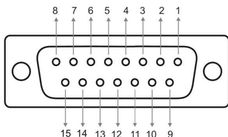
RadonixPC+ (DB15F)
